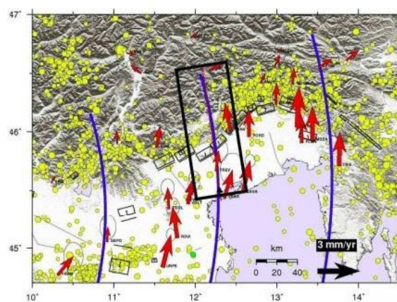
Rappresentazione schematica della cinematica della microplacca Adria in corrispondenza al margine alpino tratta da Serpelloni, 2008.
