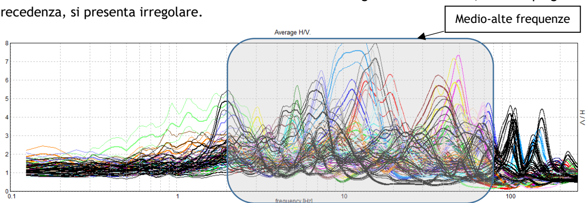
Sovrapposizione di tutte le misure H.V.S.R. condotte per il presente lavoro.
