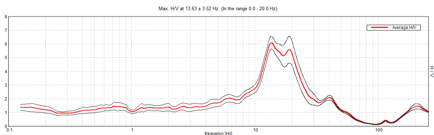
Curva H / V da misura H.V.S.R. n. 1: la curva mostra un forte contrasto sismico alle medio-alte frequenze (13,63 Hz), associabile al contatto copertura-roccia.
