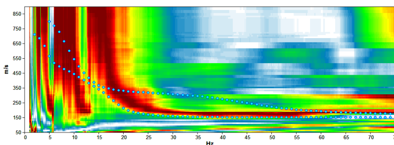
Spettro di velocità da misura sismica in array (Re.Mi. n. 18): è possibile notare l'elevata coerenza del segnale e le basse frequenze indagate.
